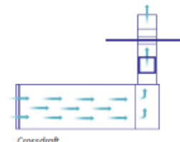
Crossdraft
